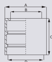
Ferrule
